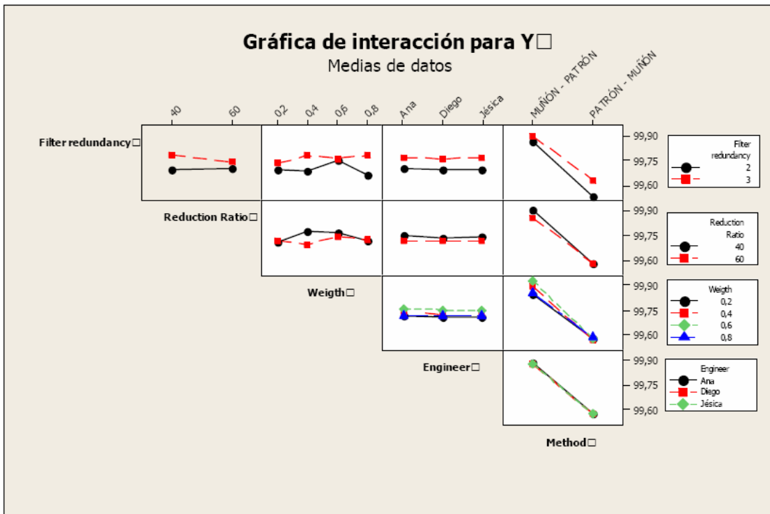
Fig. 8. Gráfica de interacción para la variable respuesta, utilizando Minitab® versión 15.
