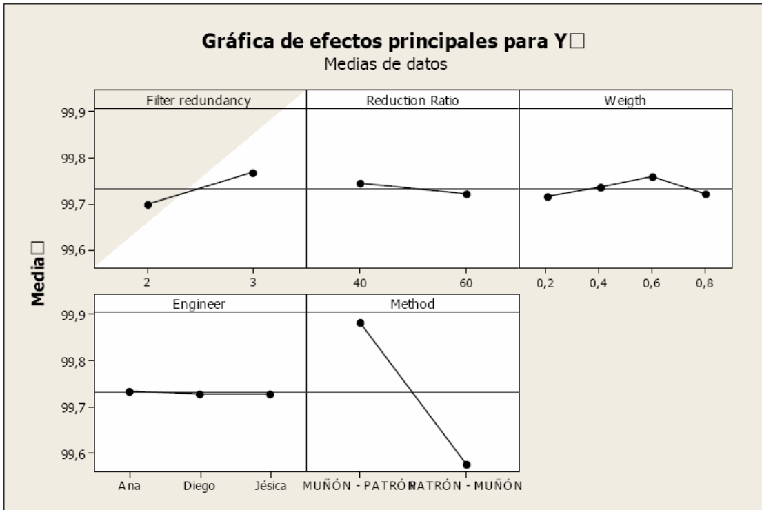
Fig. 7. Gráfica de efectos principales para la variable respuesta, utilizando Minitab® versión 15.
